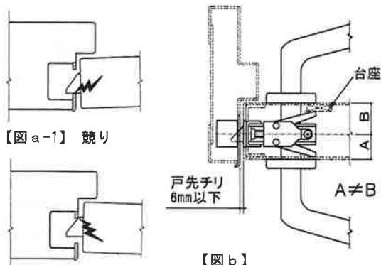
【図 a-1】 競り 【図 a-2】 オーバーラン 錠本体偏心付：振れ止め用の台座を設ける。 【図 b】
